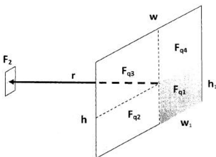
Рисунок A.3.2. Расположение излучающих поверхностей пламени F_{q1-q4} и облучаемой поверхности материала соседнего объекта F_2 , где w_1 и h_1 - длина и ширина соответствующей части поверхности пламени.
