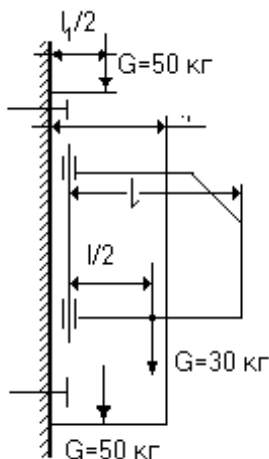
Рисунок 2. Схема приложения статической нагрузки
